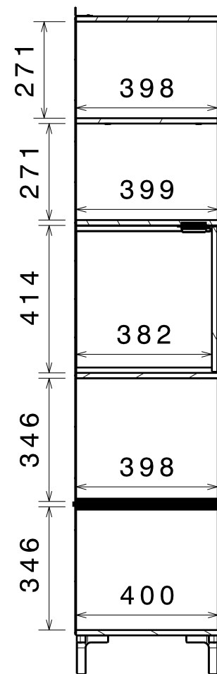
Coupe A-A
