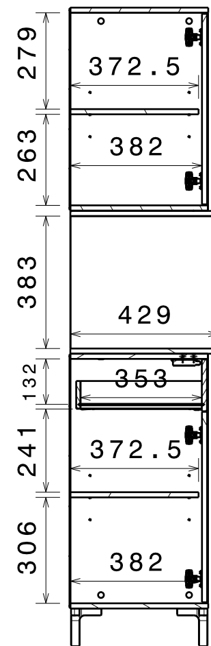
Coupe B-B
