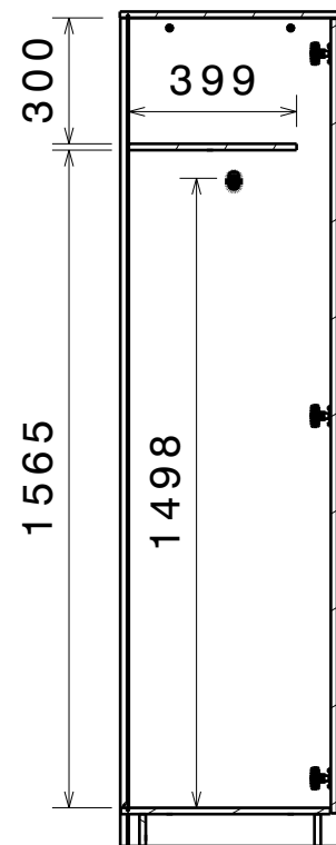
Coupe B-B
