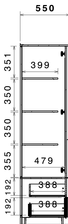
Coupe A-A
