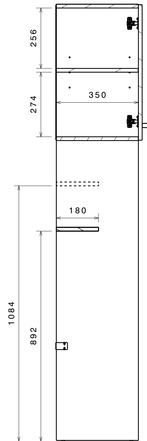
Coupe A-A Echelle : 1:10
