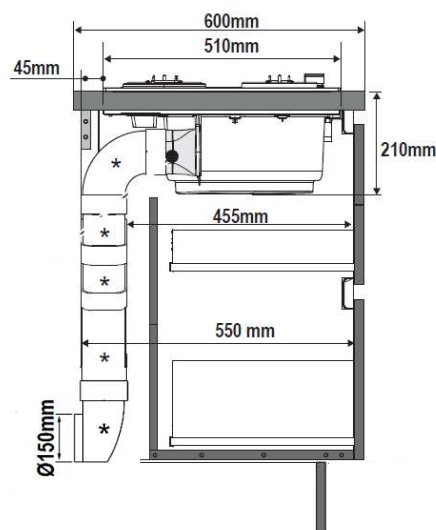
Installation directe
