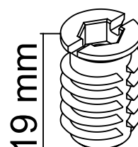
8 x Réf. 3472
